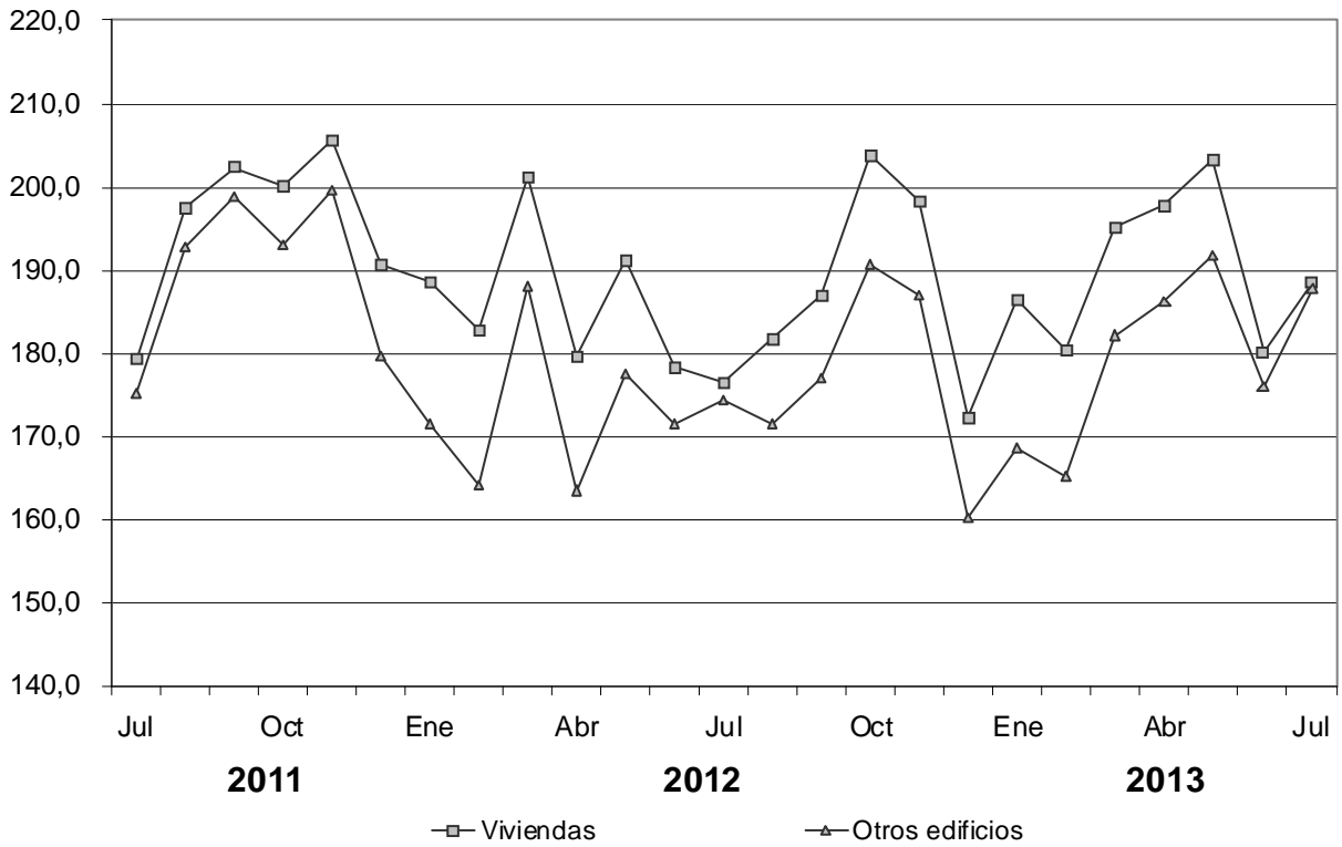
Gráfico 5. Bloques del ISAC. Edificios para viviendas y otros edificios, Julio 2011 - Julio 2013
