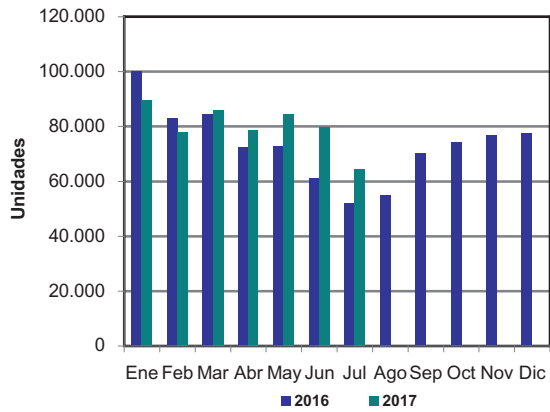
Producción de heladeras
