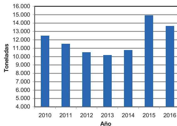
Producción de o-xileno
