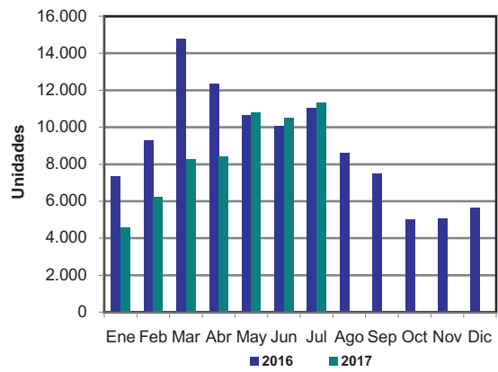
Producción de hornos y anafes
