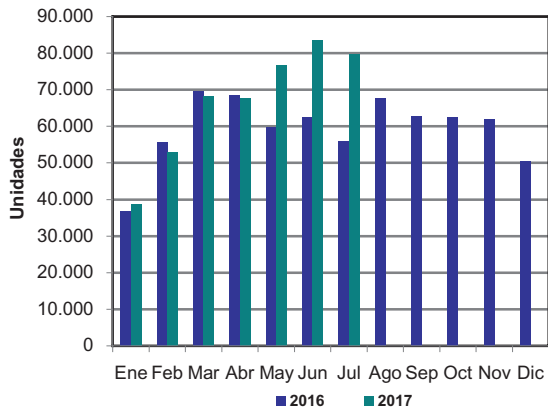
Producción de cocinas
